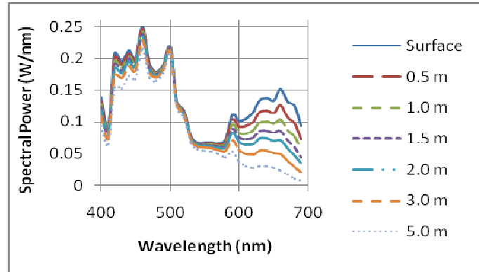
PAR Power Distribution of 10,000 K MH vs Seashine
